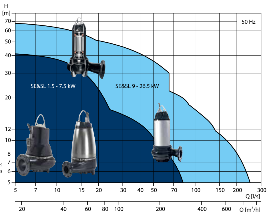
Courbes de performances des pompes SE et SL combinées
