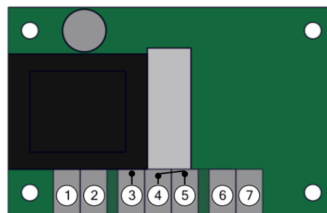
Vue intérieure de la carte électronique du Moniteur PRO3 Les contacts sont représentés au repos : moniteur en alarme ou hors tension
