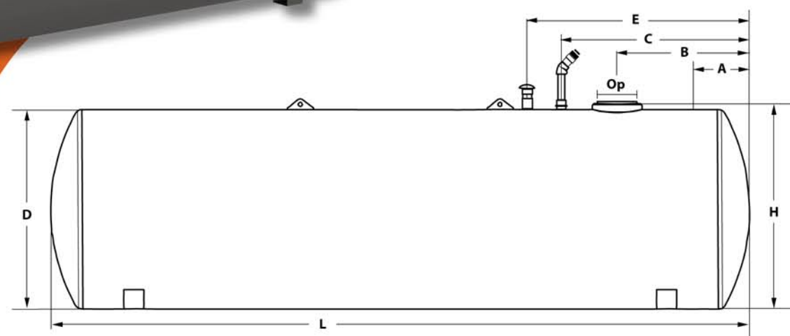
CUVE ACIER dimensions en mm et poids en kg
