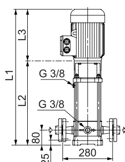
PX 8 Version standard R (acier inox 304) / N (acier inox 316) Exécution in line brides rondes
