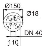
PX 8 Version standard R (acier inox 304) / N (acier inox 316) Exécution in line brides rondes
