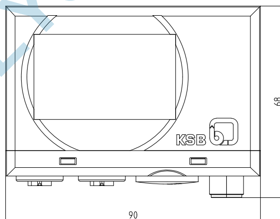
III. 10: Dimensions du module d'affichage
