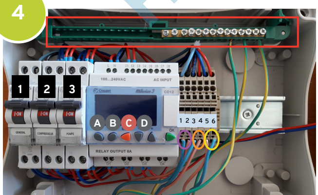
Connexion au tableau électrique.
