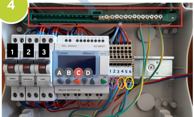
Connexion au tableau électrique.
