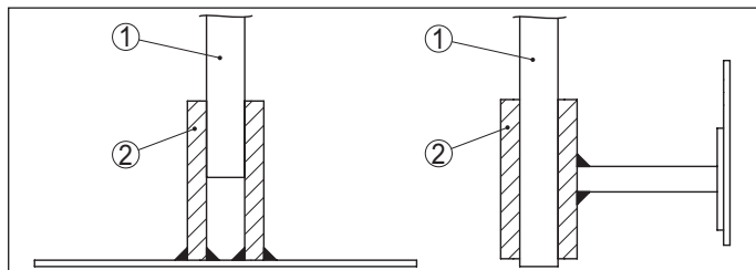
Fig. 4: Fixer la sonde de mesure
