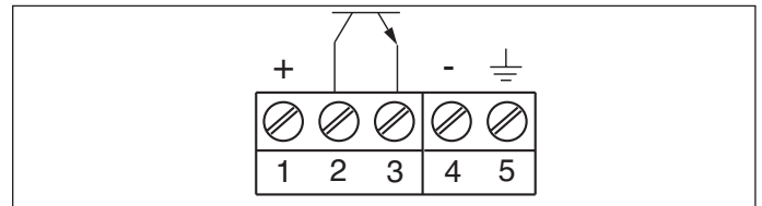
Fig. 9: VEGAKON 61 - Sortie de transistor
