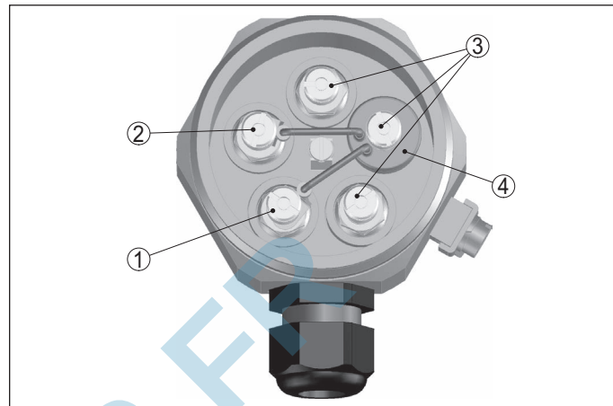
Fig. 13: Électronique supplémentaire pour la détection de circuits ouverts en liaison avec VEGATOR 131, 132
