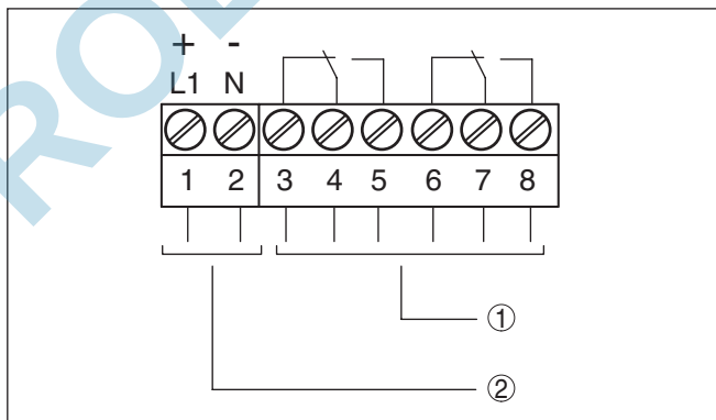
Fig. 6: Électronique avec sortie relais
