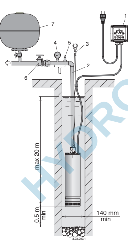
Fig. 3 Pompa sospesa Pump in the suspended position Pumpe aufgehängt Pompe suspendue Bomba suspendida Pump i upphängd position Насос в подвешенном положении 泵的悬挂安装
