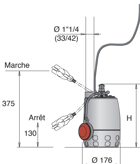
Flotteur standard
