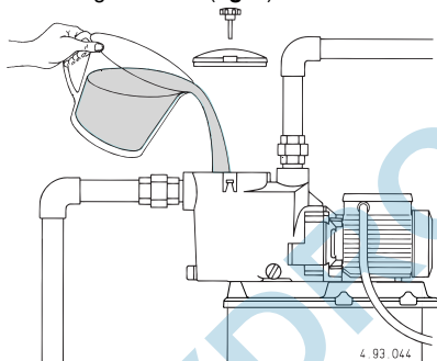
Fig. 2 Filling
