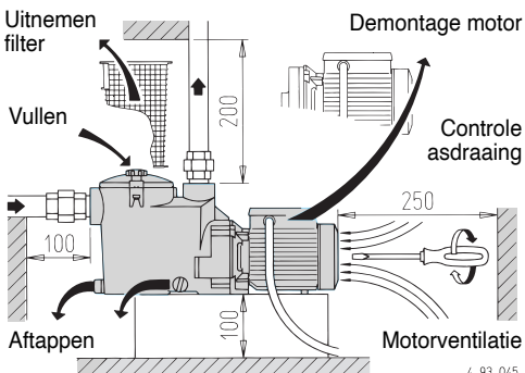
Fig. 1 Minimale ruimte voor onderhoud (mm)
