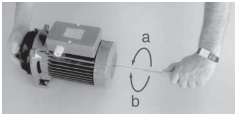
Рис. 5 Снятие (a) и установка (б) рабочего колеса.
