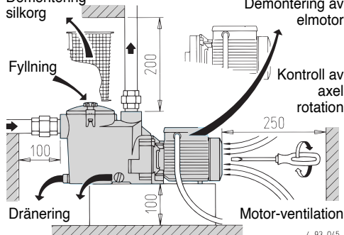
Fig. 1 Minimum utrymme för service (mm)
