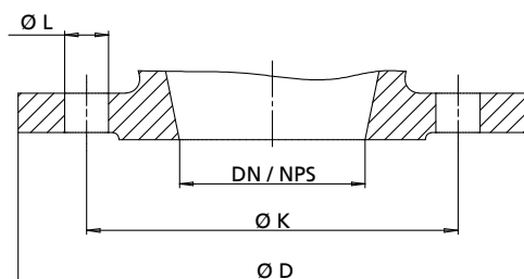
III. 5: Cotes de bridage Etaline SYT
