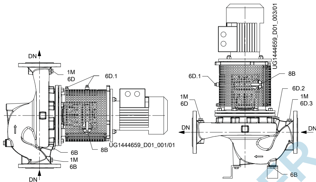
III. 4: Etaline SYT, réalisation des raccordements suivant le mode d'installation
