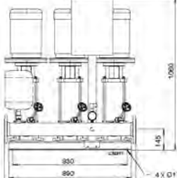
Surpresseur 3 pompes Movitec 15 en montage C-V
