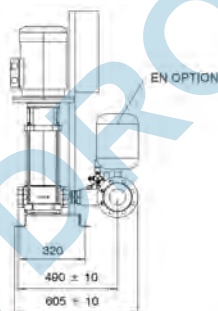
Surpresseur 3 pompes Movitec 2,4,6 et 10 en montage A
