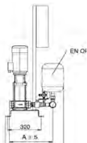
Surpresseur 3 pompes Movitec 2,4,6 et 10 en montage A
