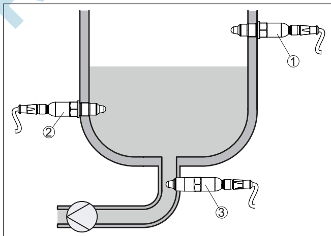
Fig. 3: Exemples de montage
