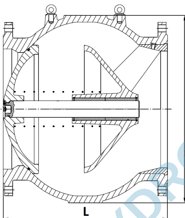
DN350 – 400
