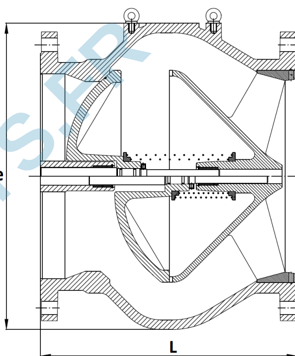
DN450 - 600
