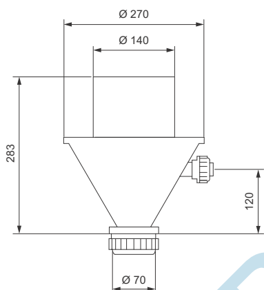
Fig. 55 Trémie de dissolution, dimensions
