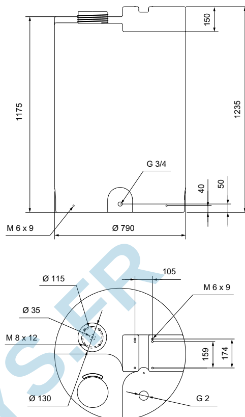
Fig. 52 Bac cylindrique, 500 litres
