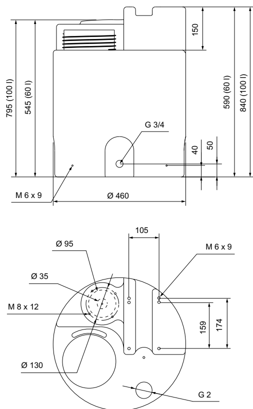
Fig. 50 Bac cylindrique, 60 et 100 litres
