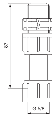
Fig. 44 Clapet de maintien de pression
