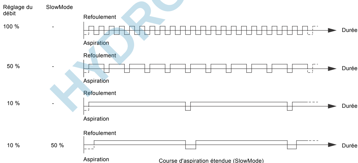
Fig. 5 Relation entre le réglage de la fréquence de course et le débit
