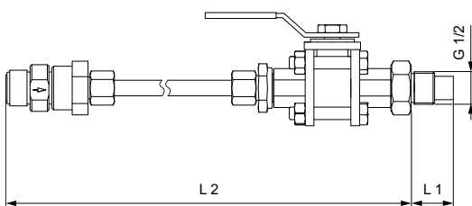
Fig. 39 Cannes d'injection d'un fluide "chaud" avec clapet à bille
