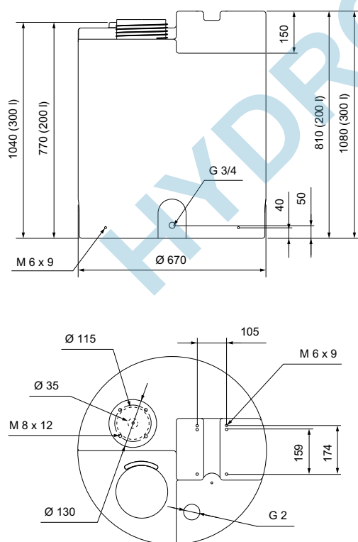
Fig. 51 Bac cylindrique, 200 et 300 litres
