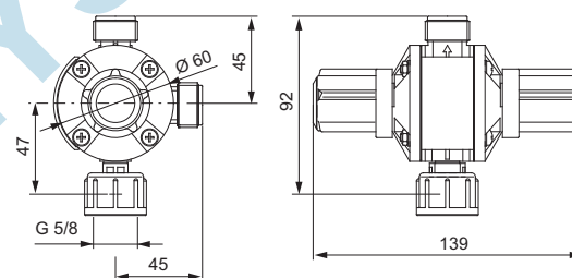
Fig. 41 Soupape multifonctions
