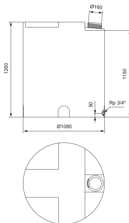
Fig. 53 Bac cylindrique, 1000 litres
