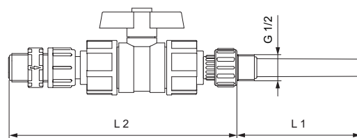
Fig. 37 Canne d'injection avec clapet à bille
