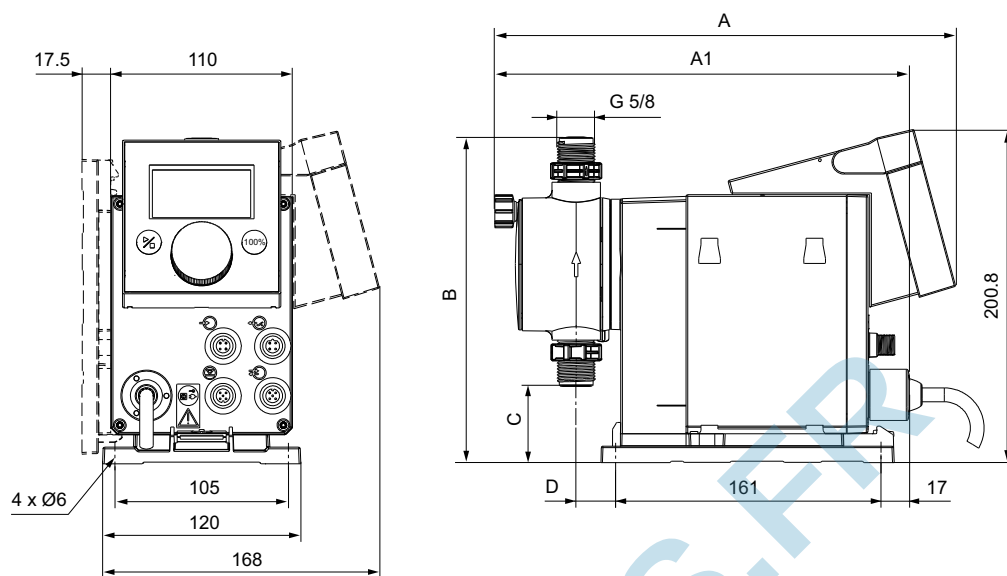
Fig. 21 DDA et DDC avec boîtier de commande monté à l'avant ou sur le côté
