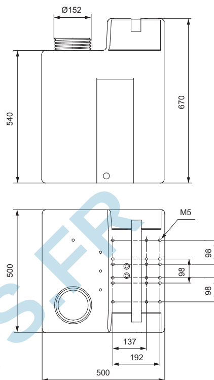
Fig. 47 Bac carré, dimensions
