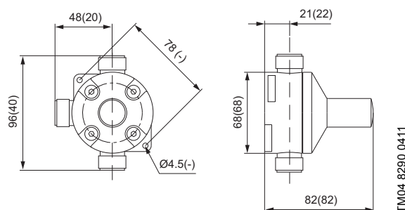
Fig. 42 Soupape de décharge. Les dimensions entre parenthèses s'appliquent au modèle inox
