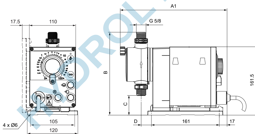
Fig. 22 DDE-PR avec éléments de commande montés en façade
