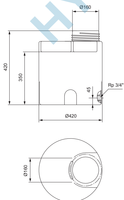
Fig. 49 Bac cylindrique, 40 litres
