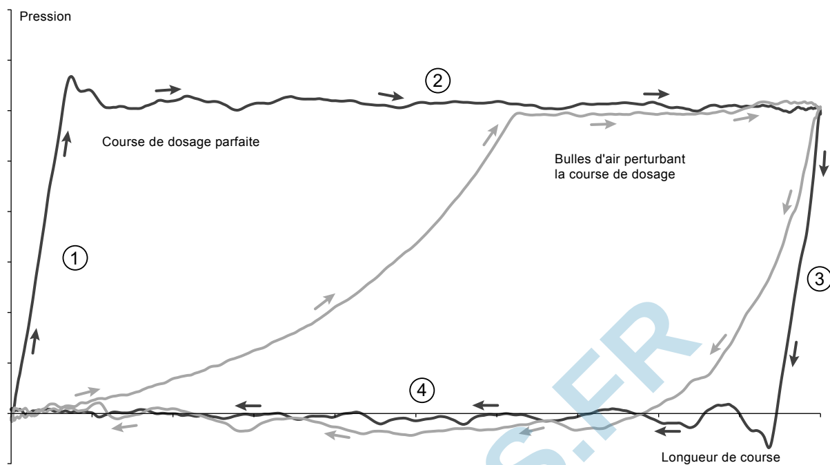
Fig. 18 Schéma
