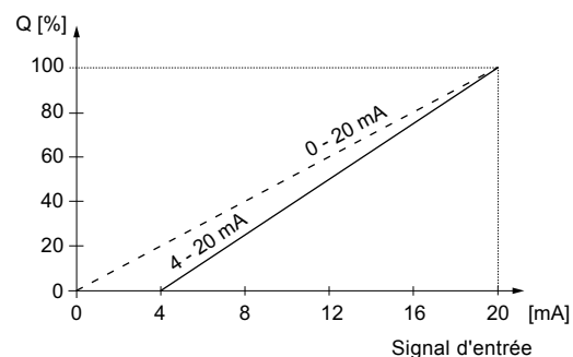
Fig. 10 Commande 0/4-20 mA
