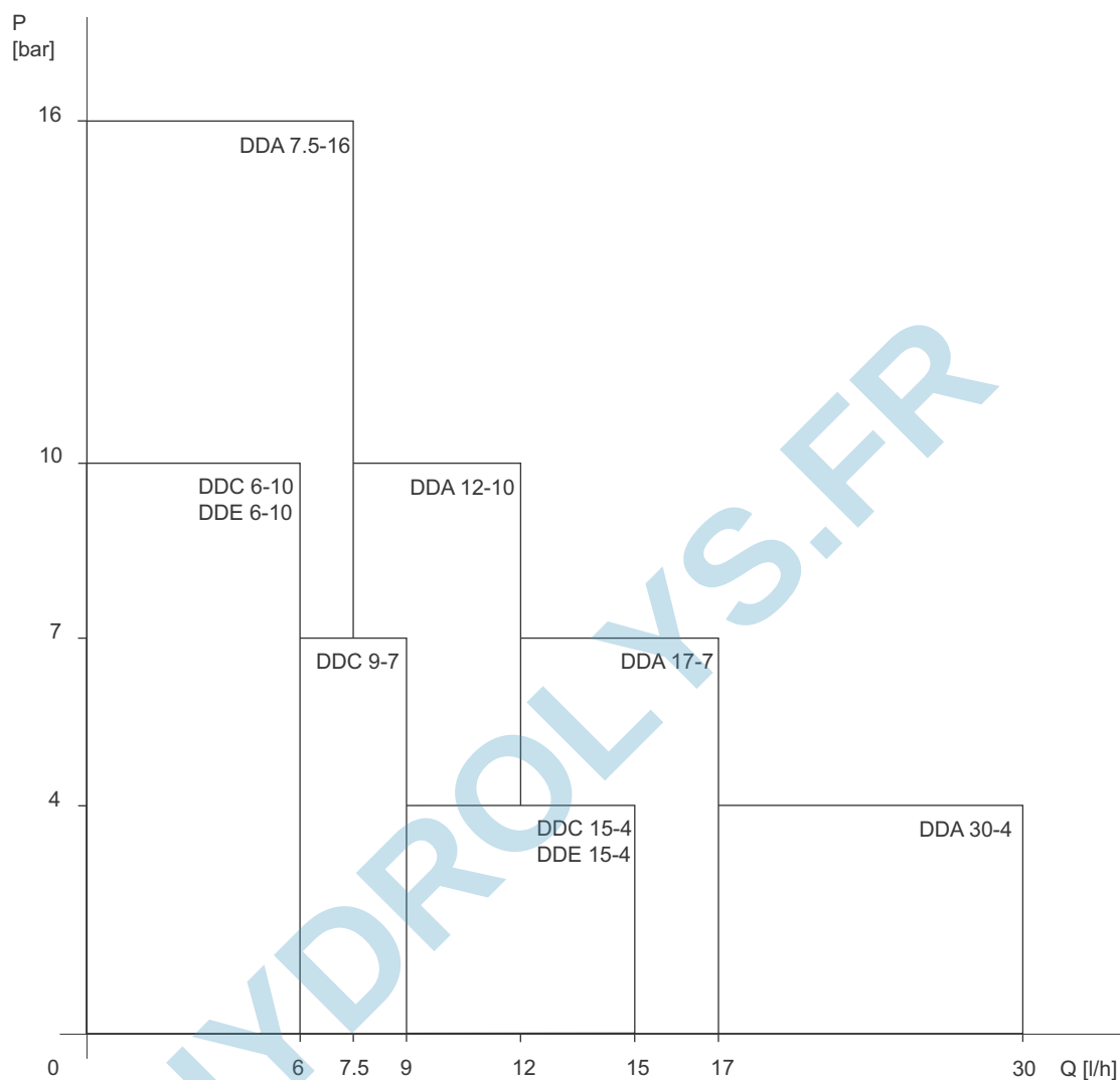
Fig. 1 Plage de performance
