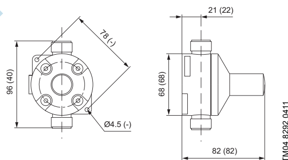
Fig. 43 Clapet de maintien de pression. Les dimensions entre parenthèses s'appliquent au modèle inox
