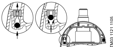
Fig. 12 Purge
