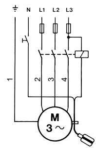
Schéma de câblage
