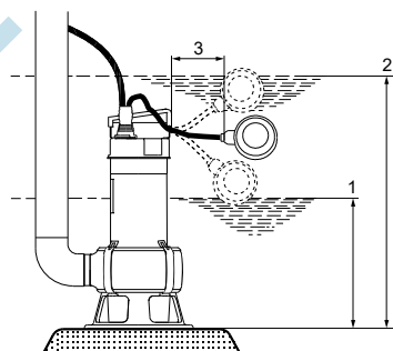
Niveaux de démarrage et d'arrêt
