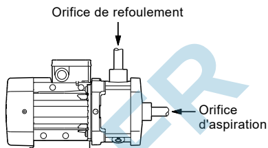
Fig. 3 Orifices d'aspiration et de refoulement
