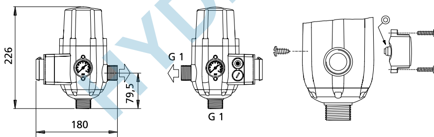
Dimensions [mm] - deux positions de montage du manomètre sont possibles.
