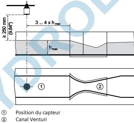
Figure 4.10 Mesure du débit avec canal Venturi Khafagi : h_{\max} = remplissage max. du canal ; B = resserrement max. du canal
