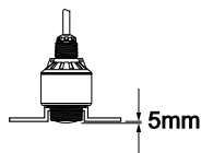
Figure 4.5 Montage recommandé du manchon fileté du SITRANS LR100
