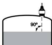
Figure 4.7 Orientation du capteur dans les liquides
