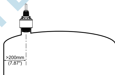
Figure 4.2 Montage du capteur radar dans une cuve à toit bombé
