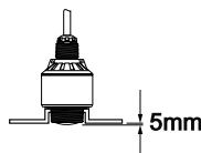
Figure 4.5 Montage recommandé du manchon fileté du SITRANS LR100
