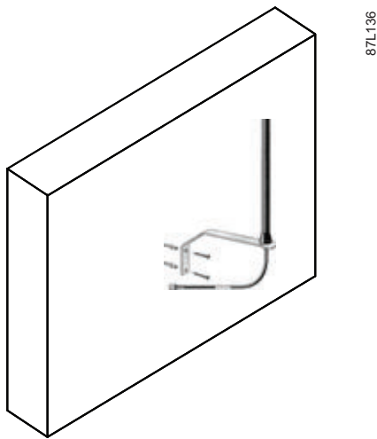
Figure 4-6 Installation d'une antenne à montage mural
