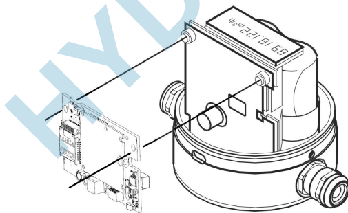
Figure 4-3 Montage du module
