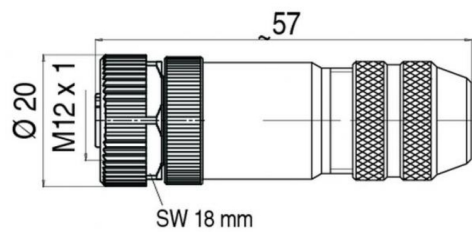
Figure 11-3 Dimensions du câble adaptateur femelle
