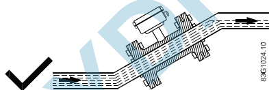
Figure 4-2 Installation correcte pour conduites remplies
