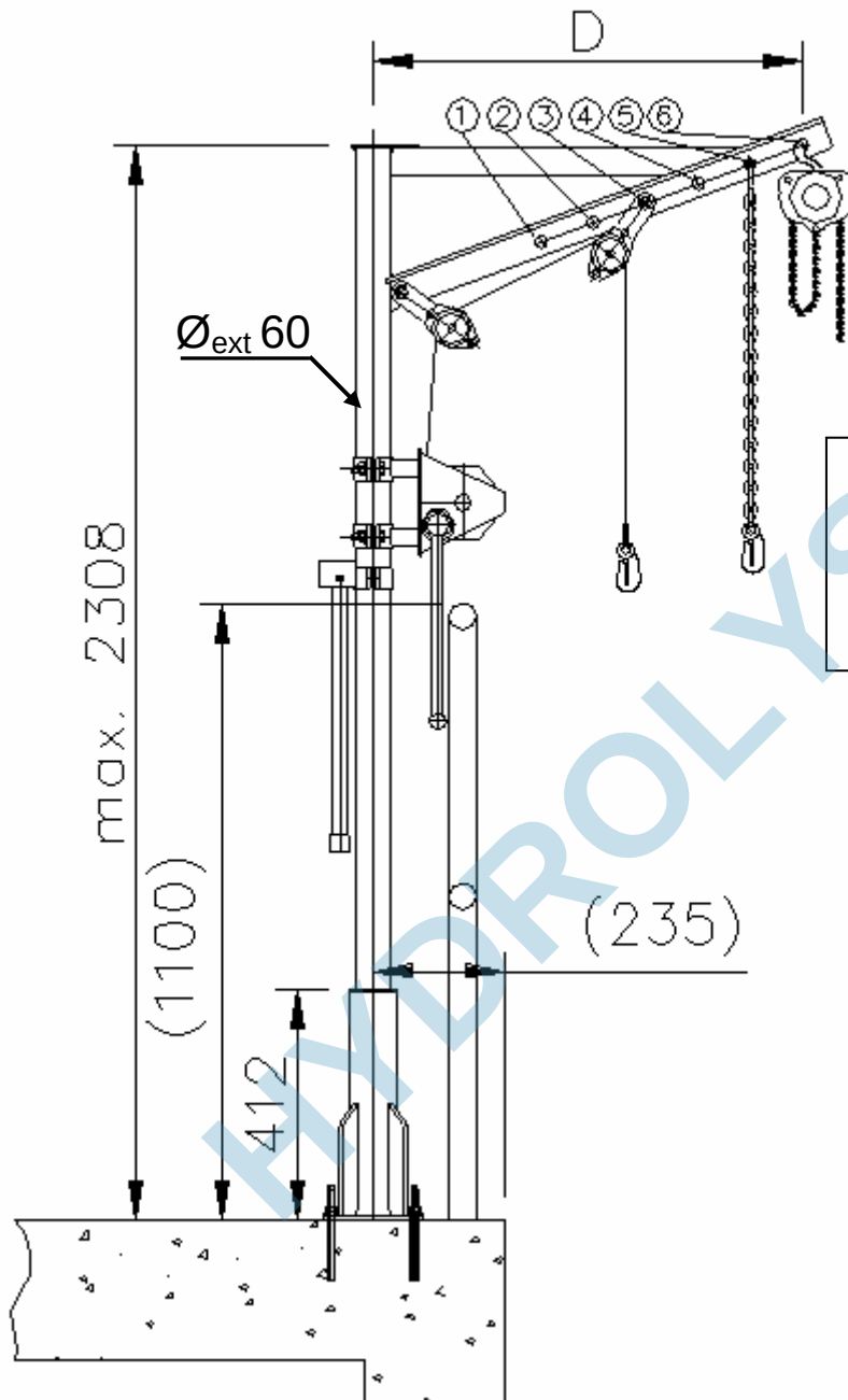
Position de la poulie en fonction de l'orientation de l'agitateur
