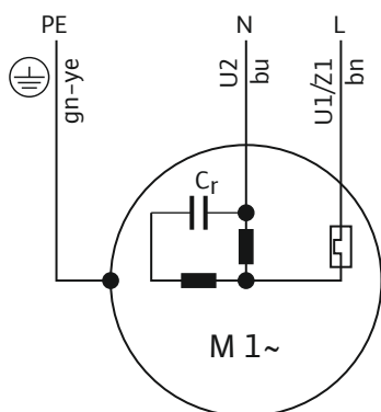
Fig. 7: Schéma de raccordement moteur 1~
