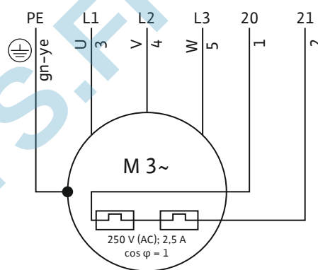
Fig. 8: Schéma de raccordement moteur 3~
