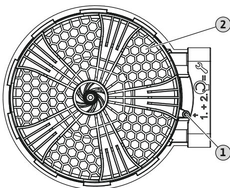
Fig. 9: Déposer le socle
