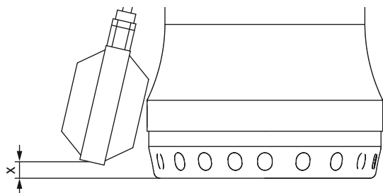
Fig. 4: Détermination de la longueur du câble du flotteur
