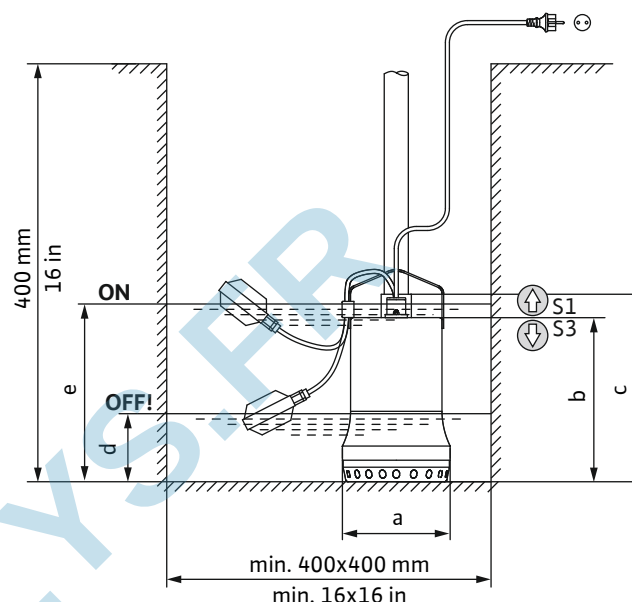
Fig. 2: Dimensions de montage et points de commutation
