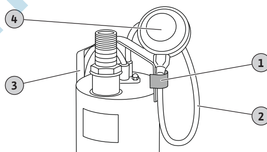
Fig. 3: Flotteur en position « Pompe Marche »
