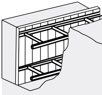
Figure 2 : étagage excavation
