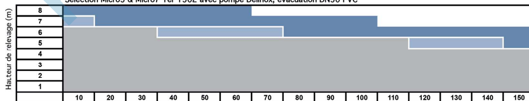
Sélection Micro5 & Micro7 Ter 1502 avec pompe Delinox, évacuation DN50 PVC
