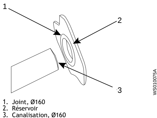
Figure 4 : Canalisation d'entrée
