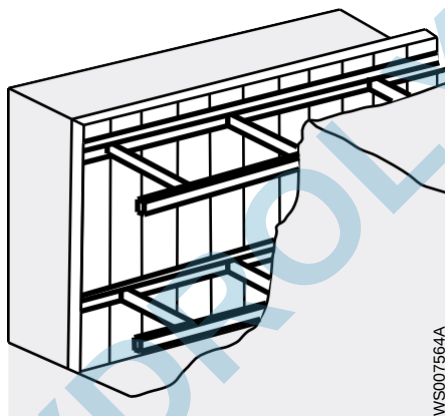
Figure 2 : Entretoisage et étréssillonage
