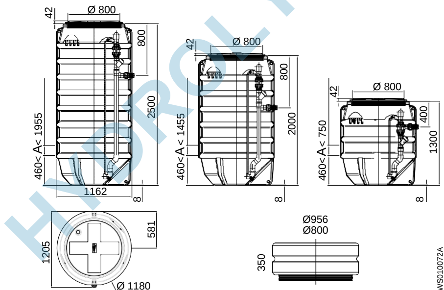
Figure 1 : Plan coté. Unité : mm
