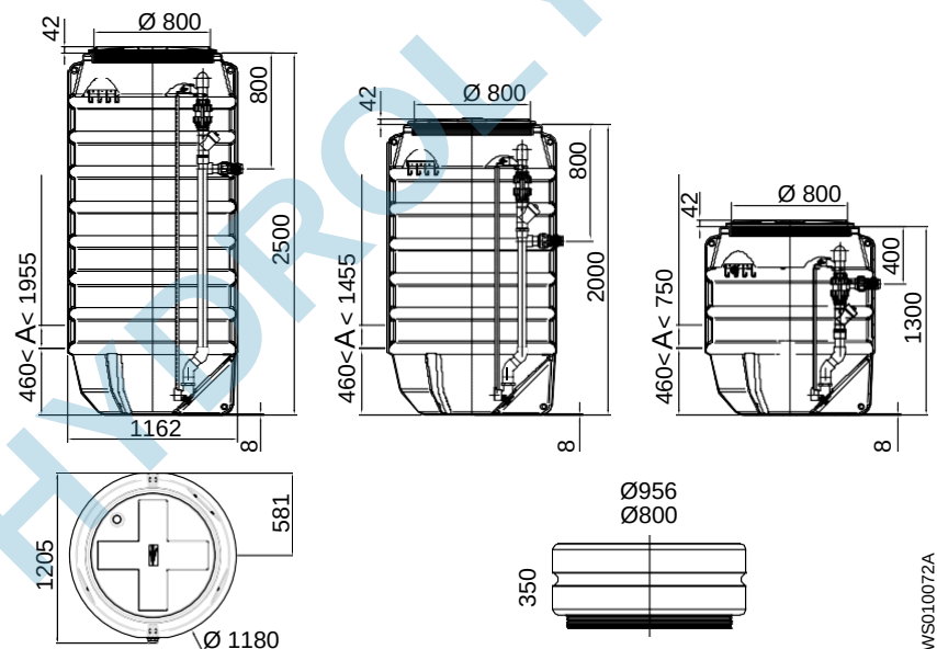
Figure 1 : Plan coté. Unité : mm
