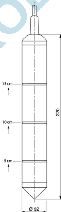
Sonde OP/..
