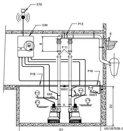
Exemple d'installation station de pompage double N 301 NE/302 NE/303 NE
