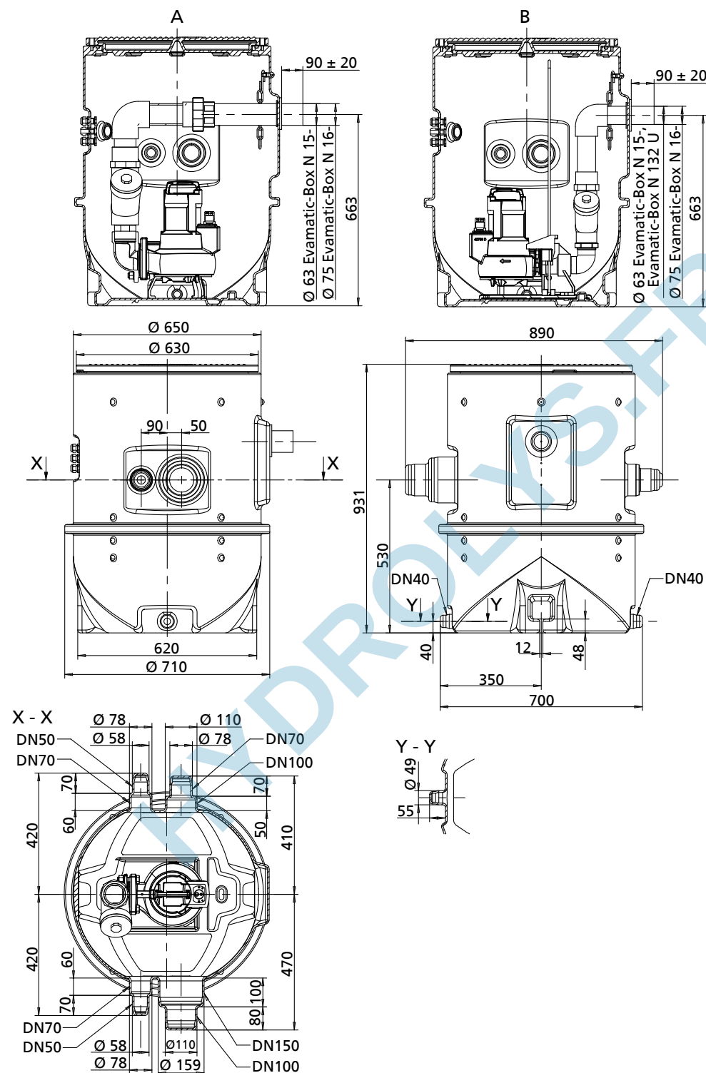
Plan d'encombrement Evamatic-Box N 200 litres
