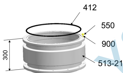
III. 3: Rehausse de couvercle
