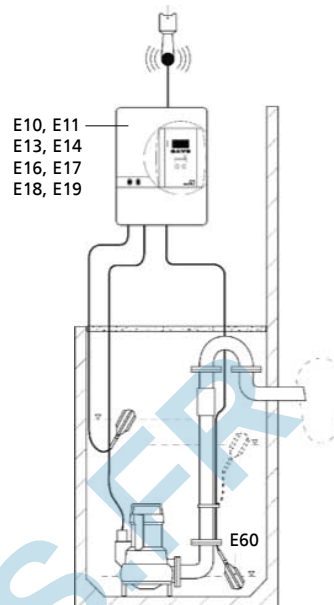
Proposition d'installation 2
