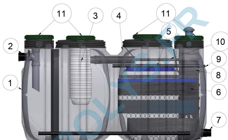
Figure 1 - Schéma de principe de la filière ACTIFILTRE® QR 2500-2500 dimensionnée pour 5 EH.
