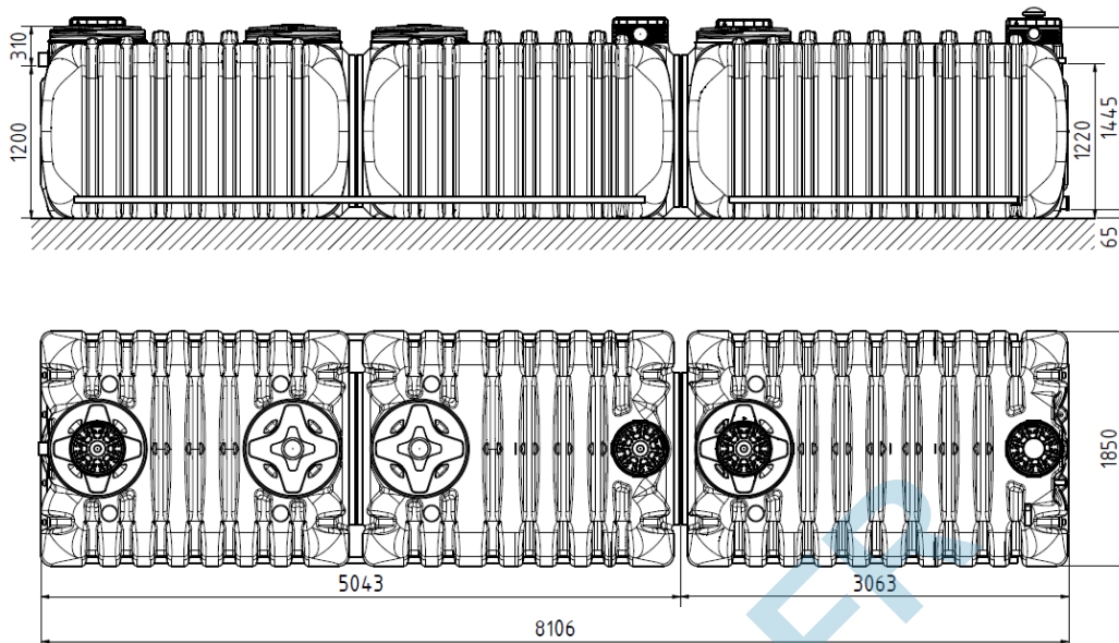
ACTIFILTRE 185 20EH
