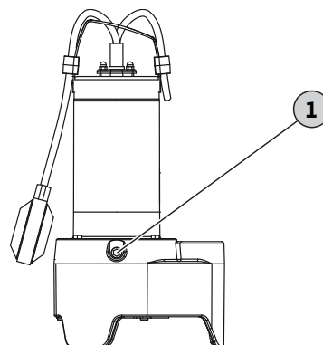
Fig. 3: Vidange d'huile de la chambre d'étanchéité
