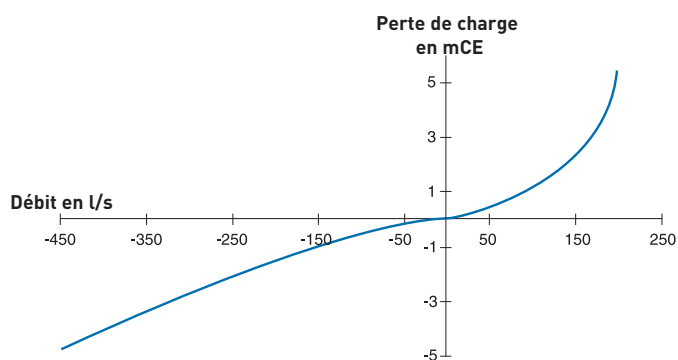
Courbe entrée/sortie d'air (large orifice)
