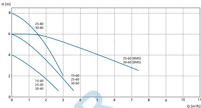
Courbes caractéristiques Calio S
