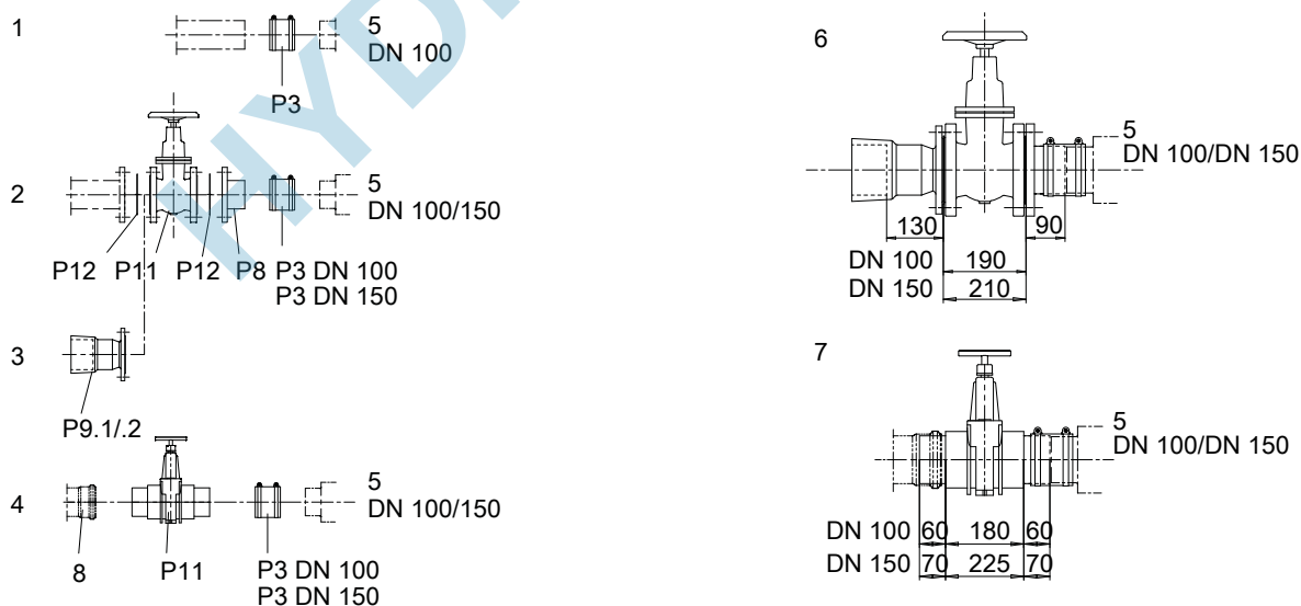
III. 33: Tuyauterie d'amenée mini-Compacta UZS (150 litres)
