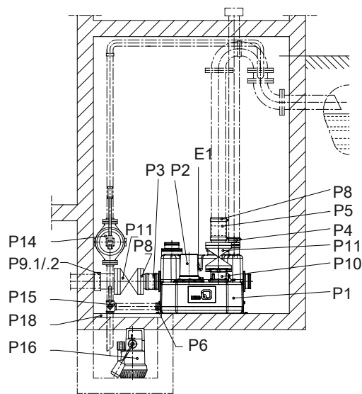
III. 26: mini-Compacta US (100 litres), représentation schématique
