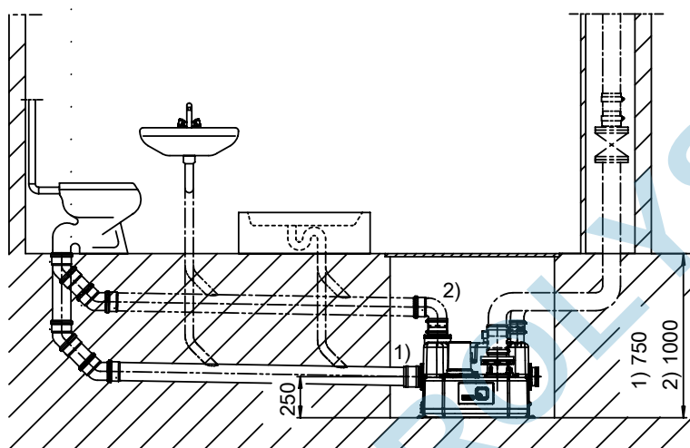
III. 16: Exemple d'installation : installation du réservoir en sous-sol, mini-Compacta US40 / U60 / U100 / US100
