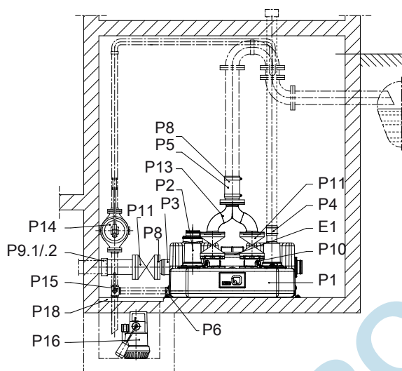
III. 32: mini-Compacta UZS (150 litres), représentation schématique
