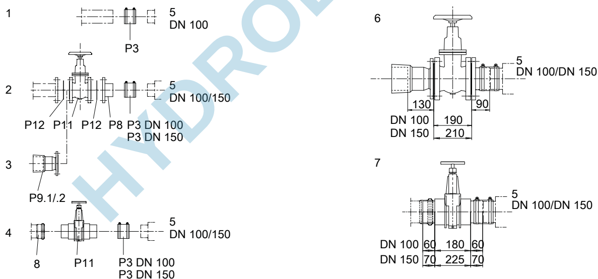
III. 24: Tuyauterie d'amenée mini-Compacta U (100 litres)
