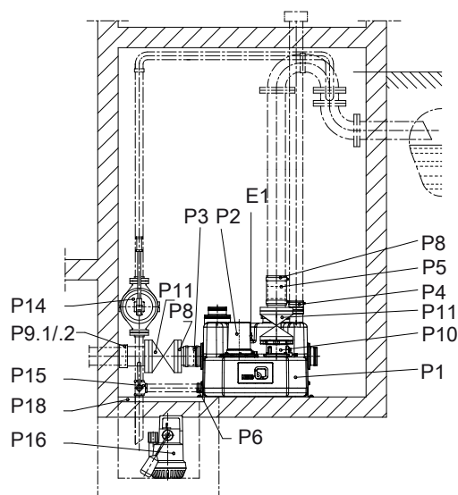
III. 17: mini-Compacta US (40 litres), représentation schématique
