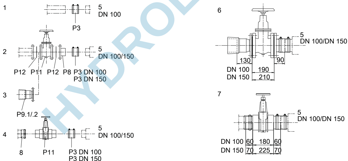
III. 21: Tuyauterie d'amenée mini-Compacta U (60 litres)
