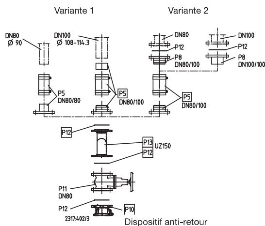
mini-Compacta U60, U100, UZ150 Conduite de refoulement
