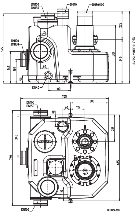
mini-Compacta U60
