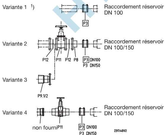
mini-Compacta U60, U100, UZ150 Conduite d'amenée
