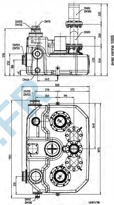
mini-Compacta UZ150
