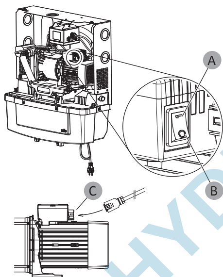
Fig. 23: Ein-/Ausschalter und Anschluss Stromversorgung
