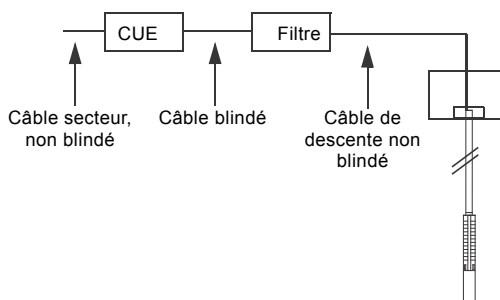
Fig. 23 Exemple d'installation sur sites non soumis aux interférences CEM
