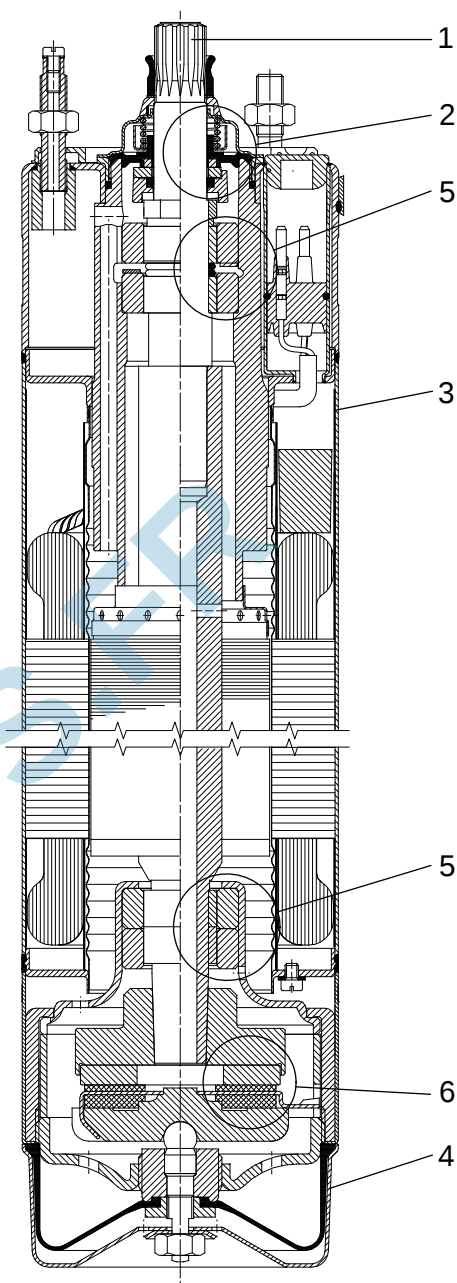
Fig. 16 MS 4000
