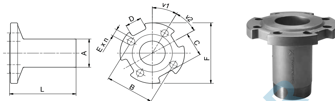
Fig. 30 Schéma coté et photo du raccord filetage-bride
