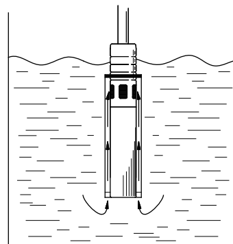
Fig. 34 Rôle de la chemise de refroidissement
