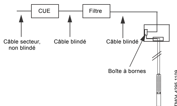
Fig. 24 Exemple d'installation sur sites soumis aux interférences CEM
