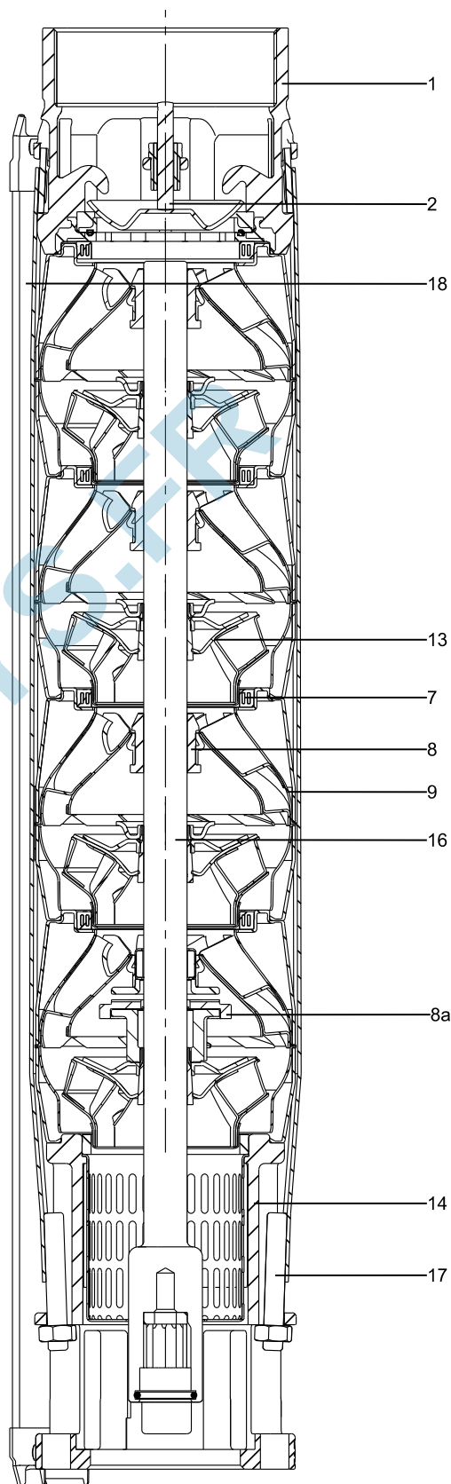
Fig. 10 Exemple SP 46
