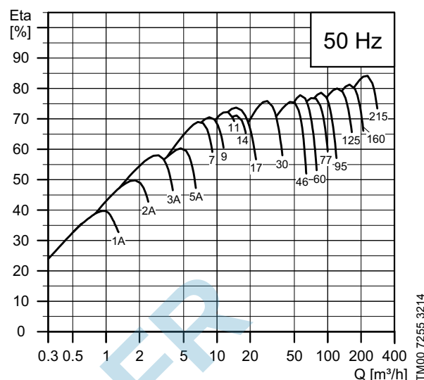
Fig. 1 Rendement pompe/moteur par rapport au débit
