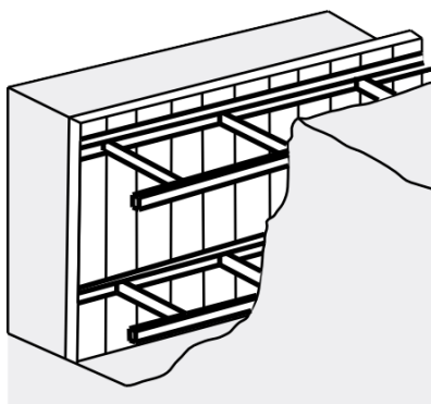
Figure 2 : étagage excavation
