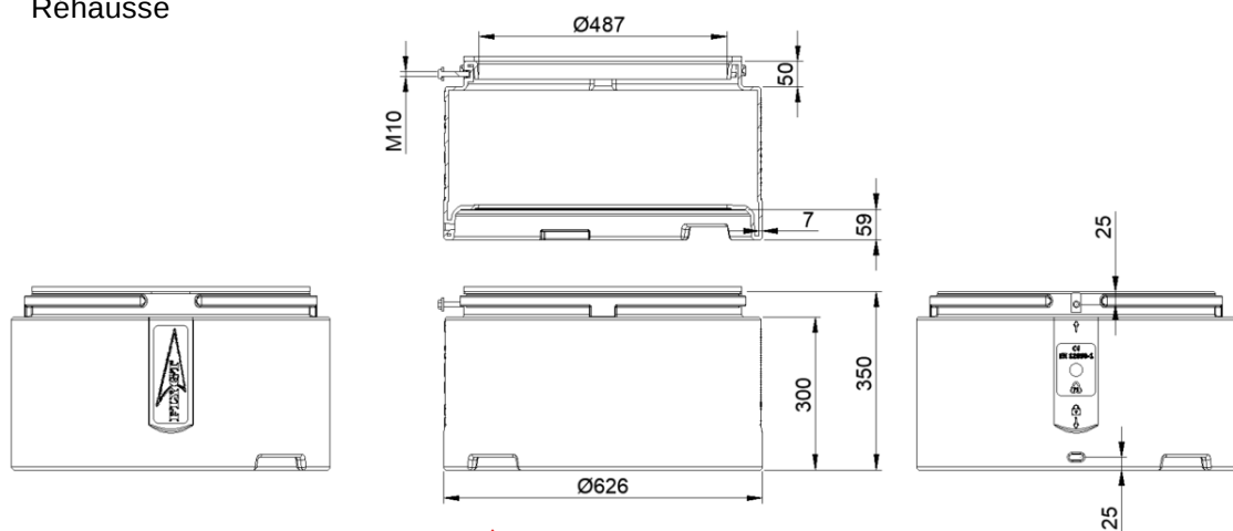
Couvercle
