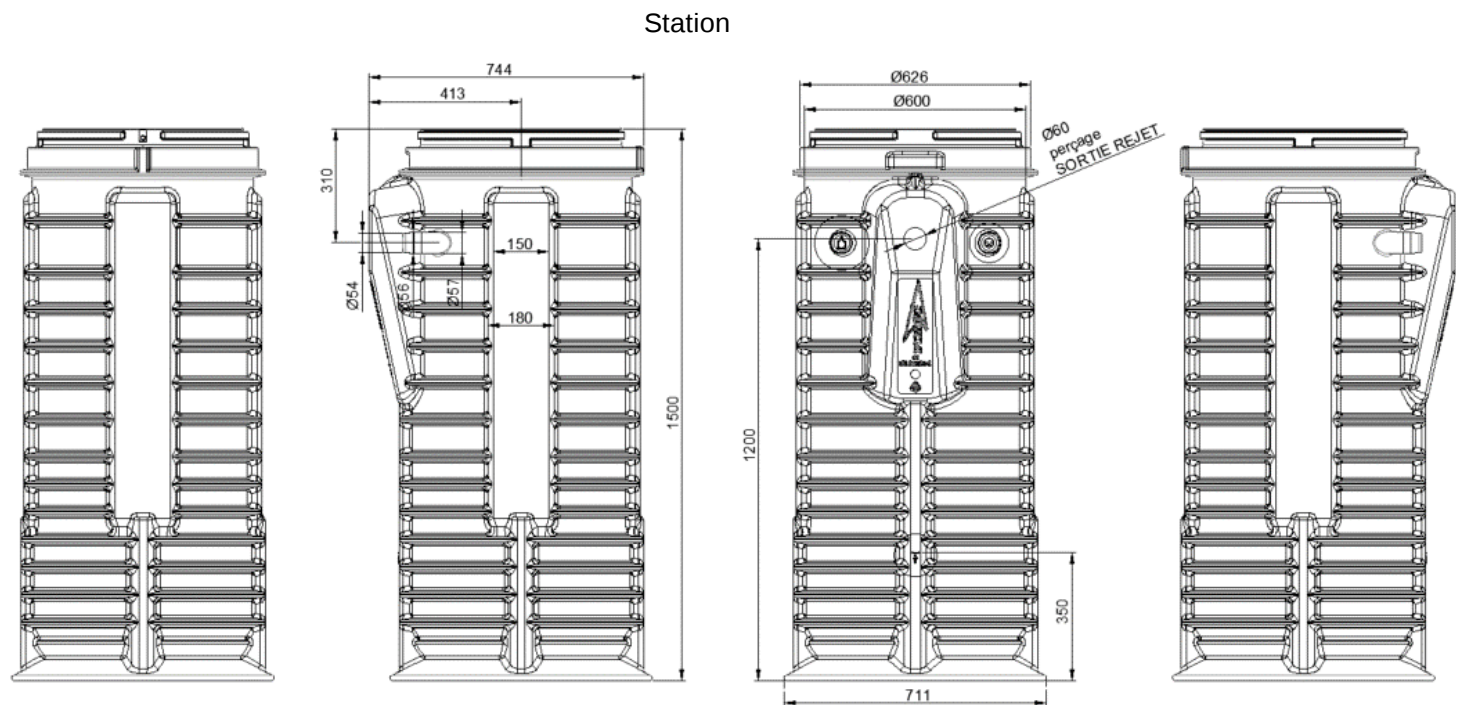
Réhausse
